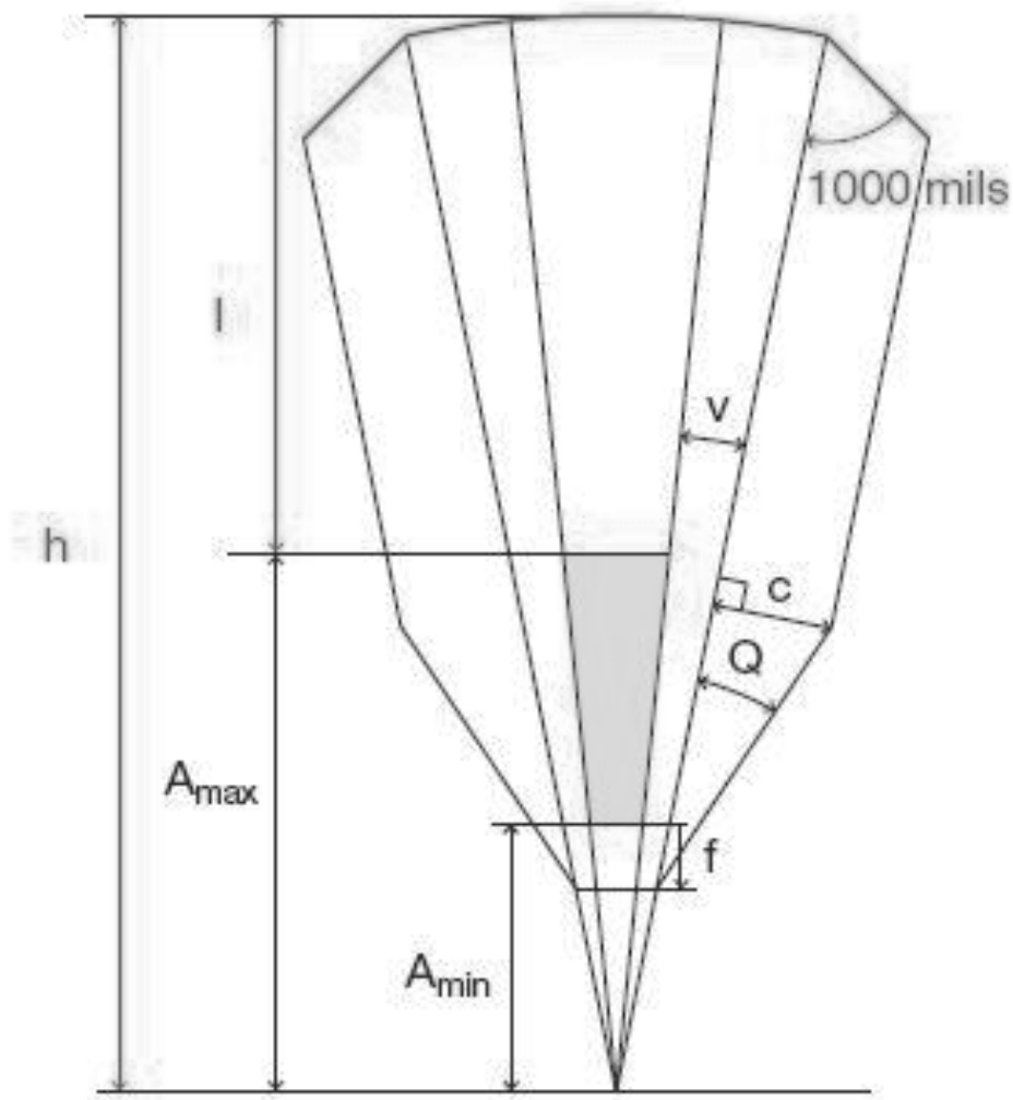
BILD 4: A Exempel på riskområde
