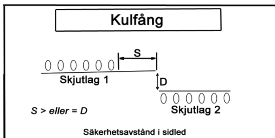
Bild 2: C Säkerhetsavstånd i sidled vid skjutning med pistol
